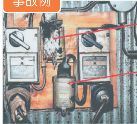
焼損したコンデンサ
